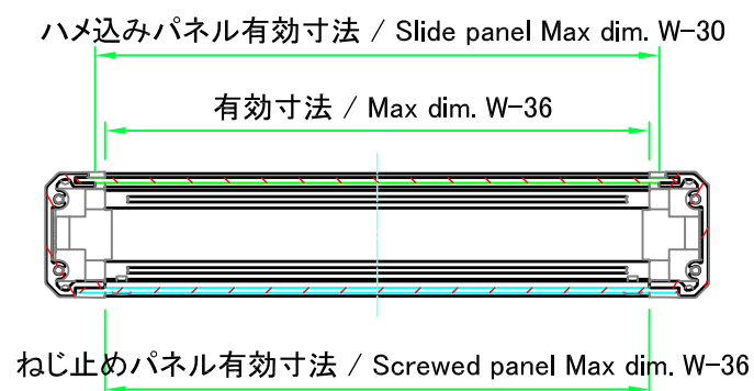
A-A ( 1 : 2.5 )
